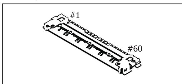
20525-060E-01(I-PEX)
