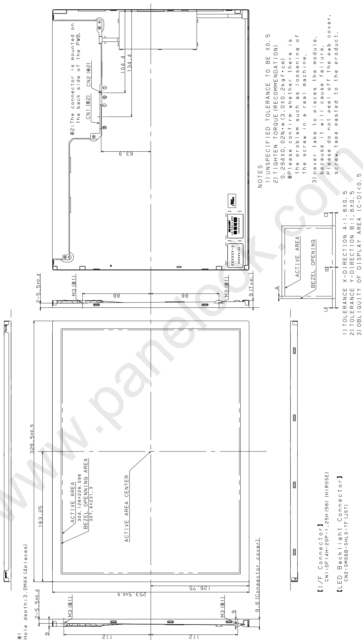
图1. LQ150X1LW95外形尺寸图
