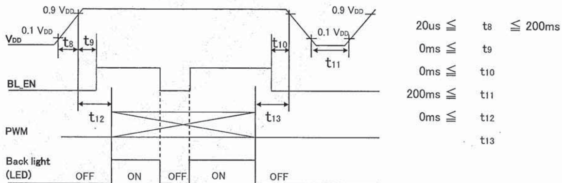
【Note1】 入力電圧シーケンス On-off conditions for supply voltage
