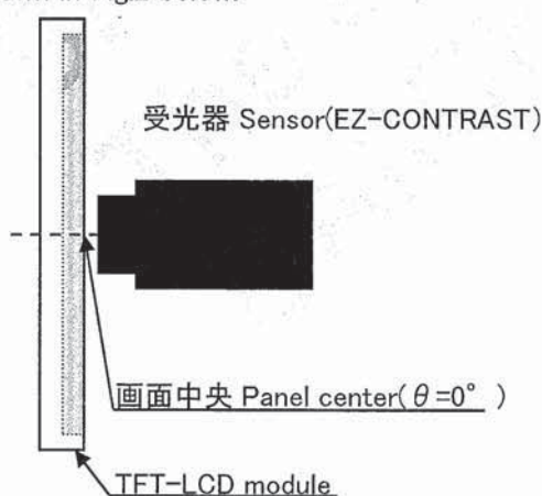
図2-1 視野角特性測定方法
